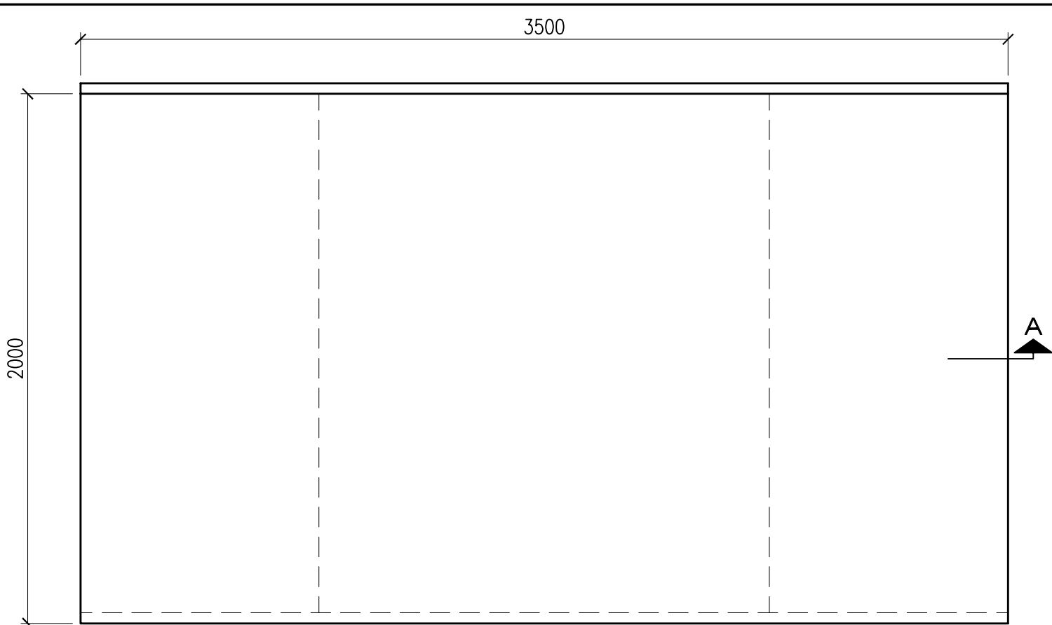
ELEVATION
